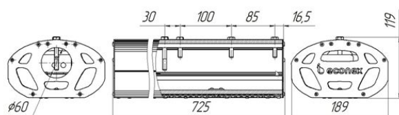
Рисунок 1. Econex Road 80/100/140/160 G2
