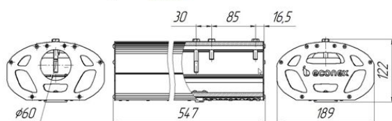
Рисунок 2. Econex Road 90/120 G2
