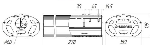
Рисунок 4. Econex Road 25 G2
