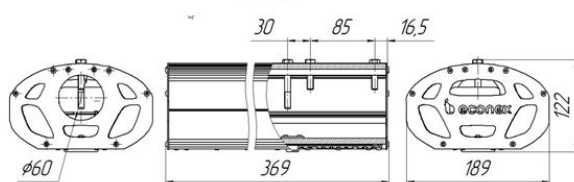
Рисунок 3. Econex Road 40/50/60/70 G2
